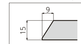
断面形状
