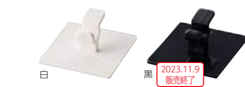
1901 白 黒 キャッチャー (受け) 40×40×18 ¥60×20P プラスチック 2023.11.9 販売終了
