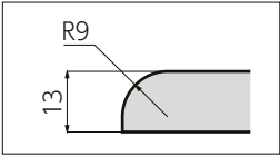
断面形状
