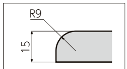
断面形状
