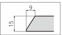
断面形状
