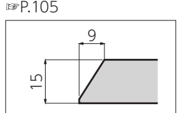
断面形状
