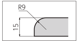
断面形状
